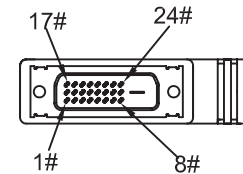
DVI(24+1)MALE
