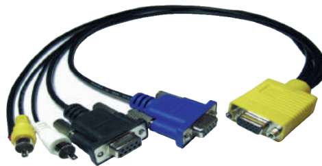
■ HD15 F to 2*DB9 F+2*RCA M + OPEN
